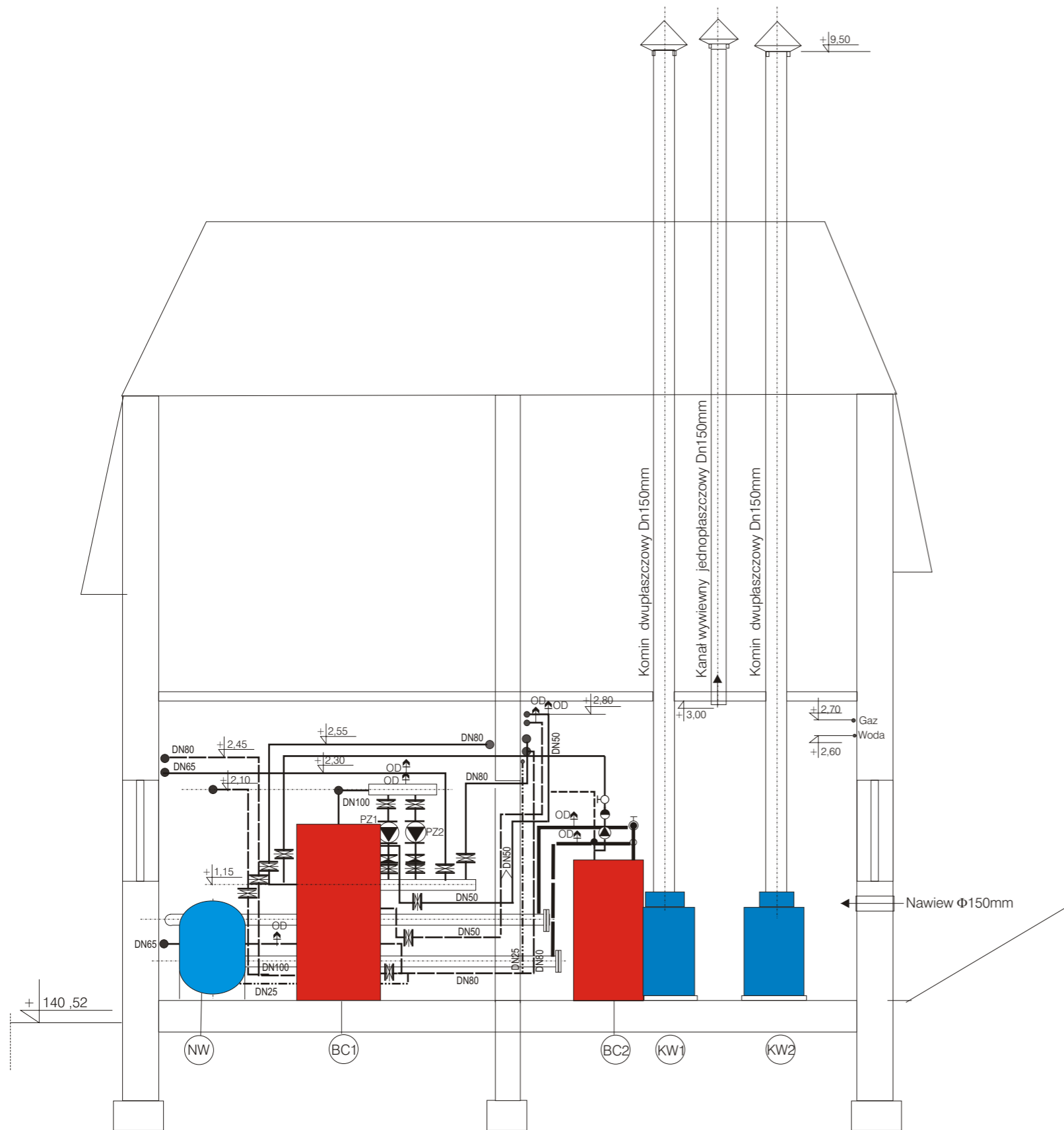
PRZEKRÓJ C - C SKALA 1 : 100 INSTALACJE CIEPLNE TECHNOLOGICZNE ŹRÓDŁA CIEPŁA
